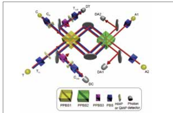
今回実現した光量子回路。光子1個レベルで動作するスイッチを組み合わせることで光量子コンピューターの基本となる量子ゲート操作を実現。
